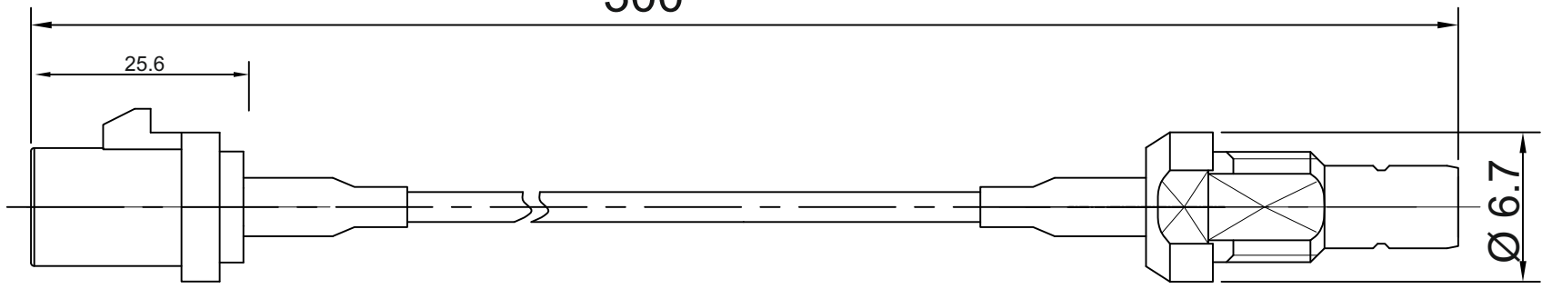
SMB plug
